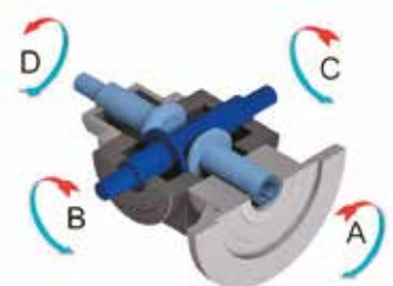
Rotazioni forma costruttiva TIPO 16 TYPE 16 constructive form revolutions
