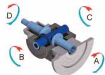
Rotazioni forma costruttiva TIPO 20 TYPE 20 constructive form revolutions
