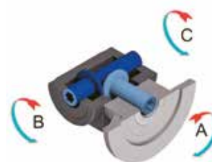
Rotazioni forma costruttiva TIPO 15 TYPE 15 constructive form revolutions
