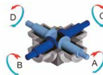
Rotazioni forma costruttiva TIPO 31 TYPE 31 constructive form revolutions
