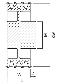
4A forme disque avec trous
