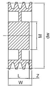
5A forme disque avec trous
