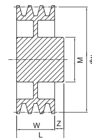
4 forme disque avec trous
