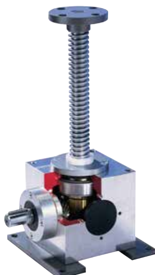
Vérin à vis grande vitesse SHG G 25 dans un boîtier en aluminium
